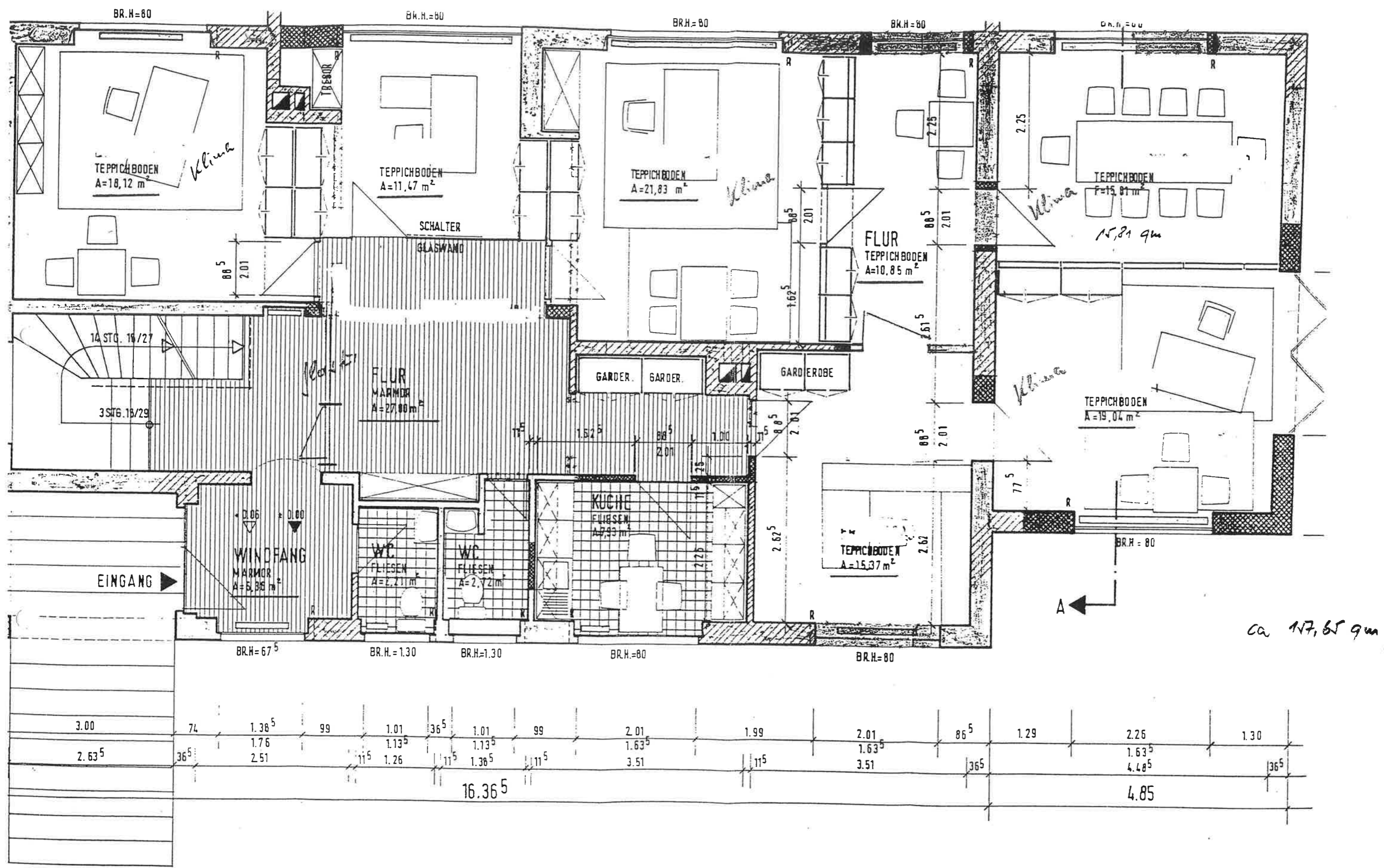
1. OGESCHOSS - GRUNDRISS
