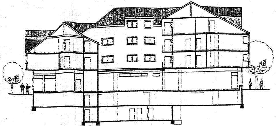
Gebäudeschnitt
