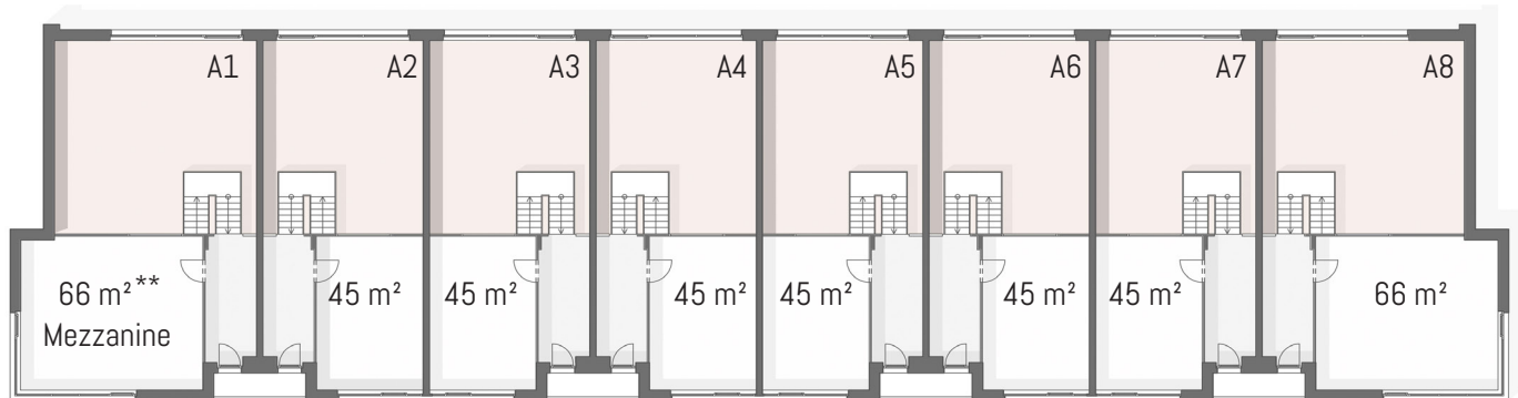
Grundriss Obergeschoss
