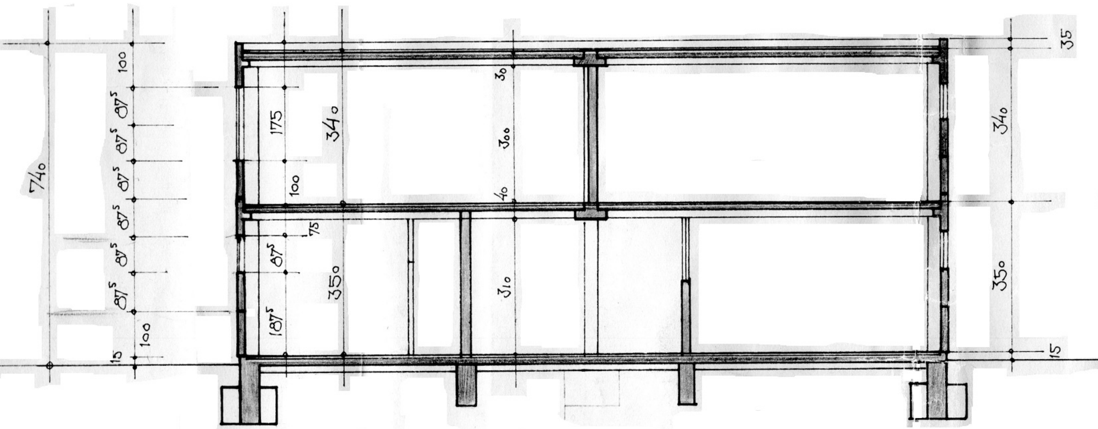
SCHNITT A - B
