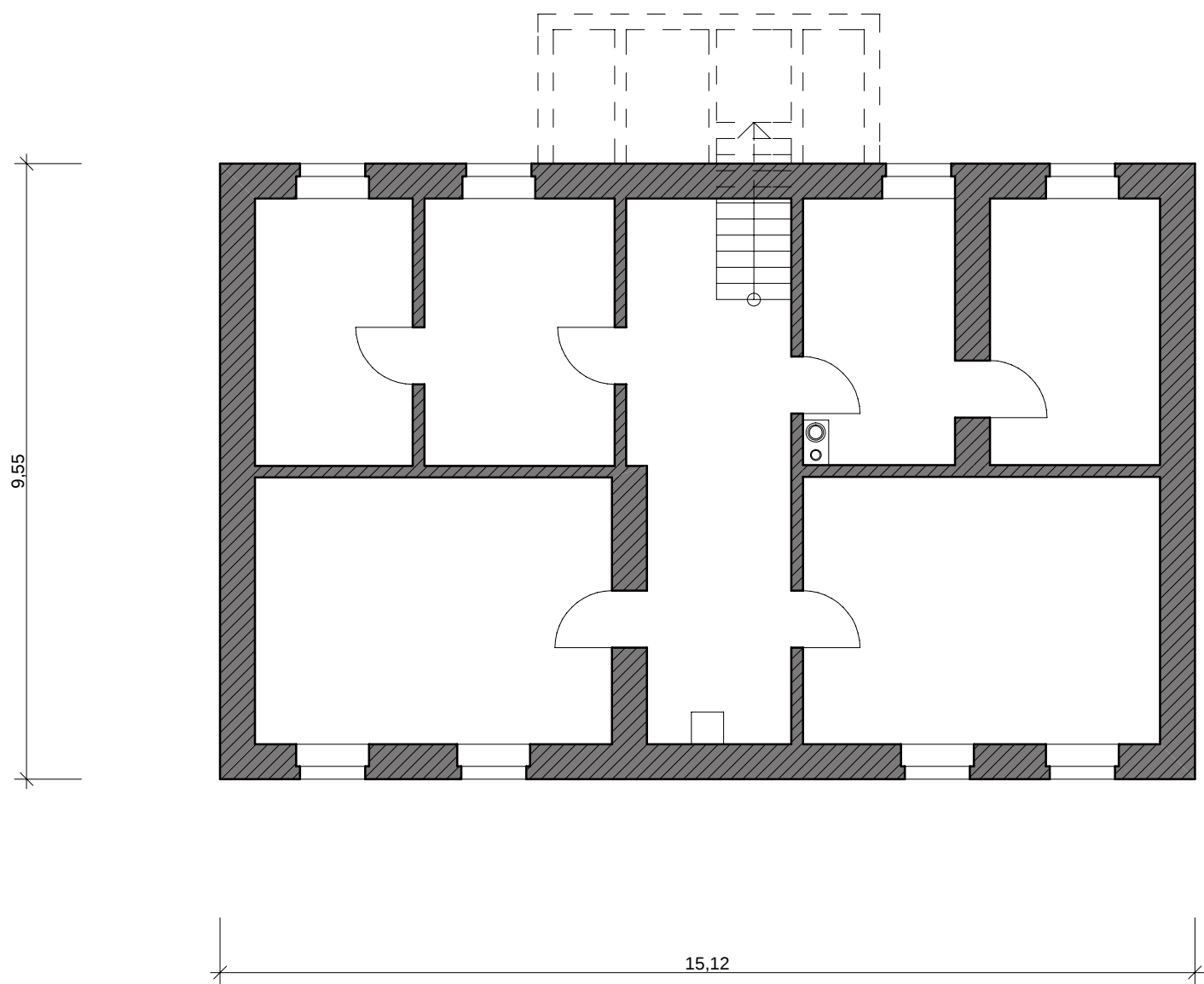
Grundriss Kellergeschoss
