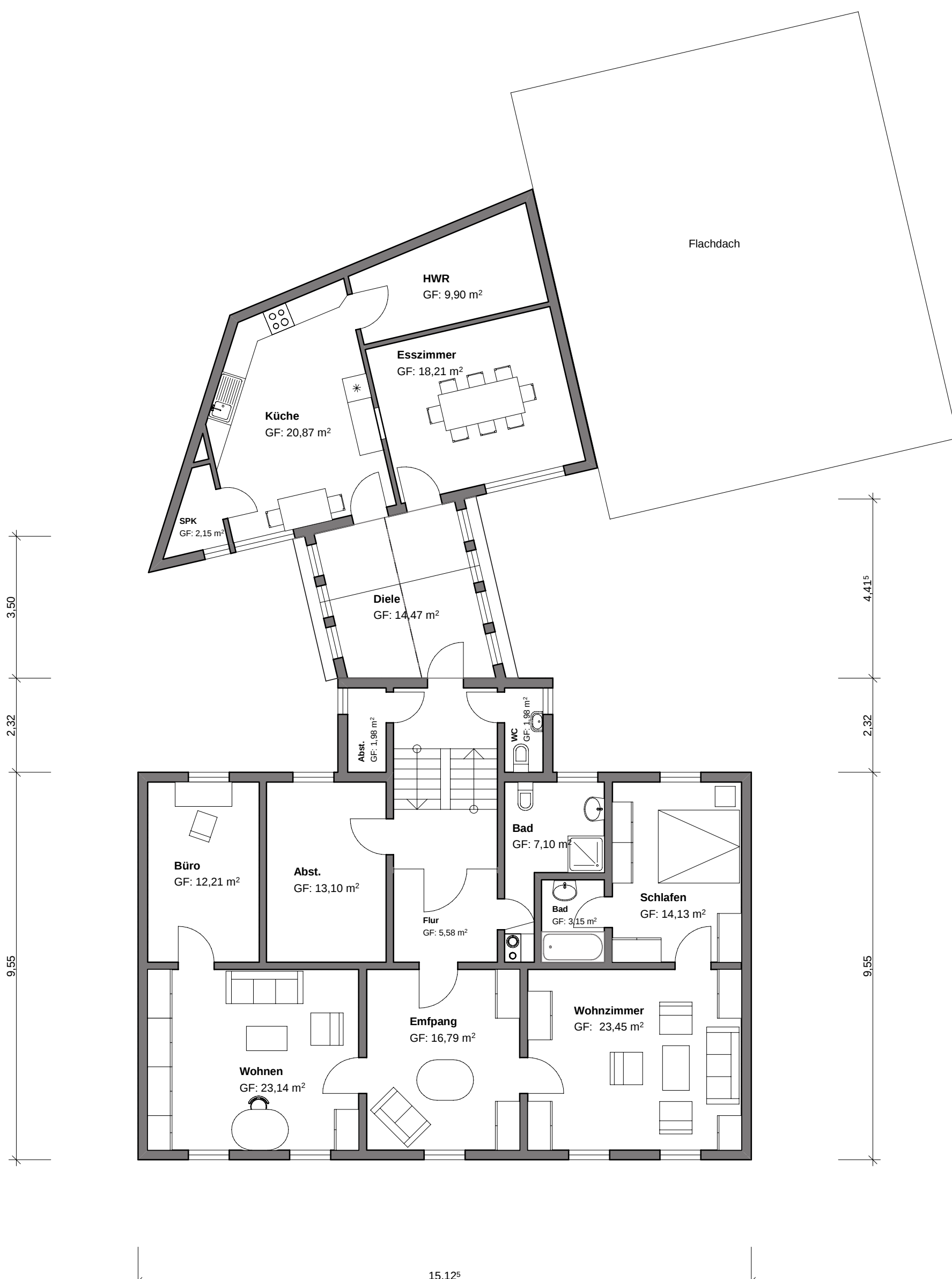
Grundriss Obergeschoss
