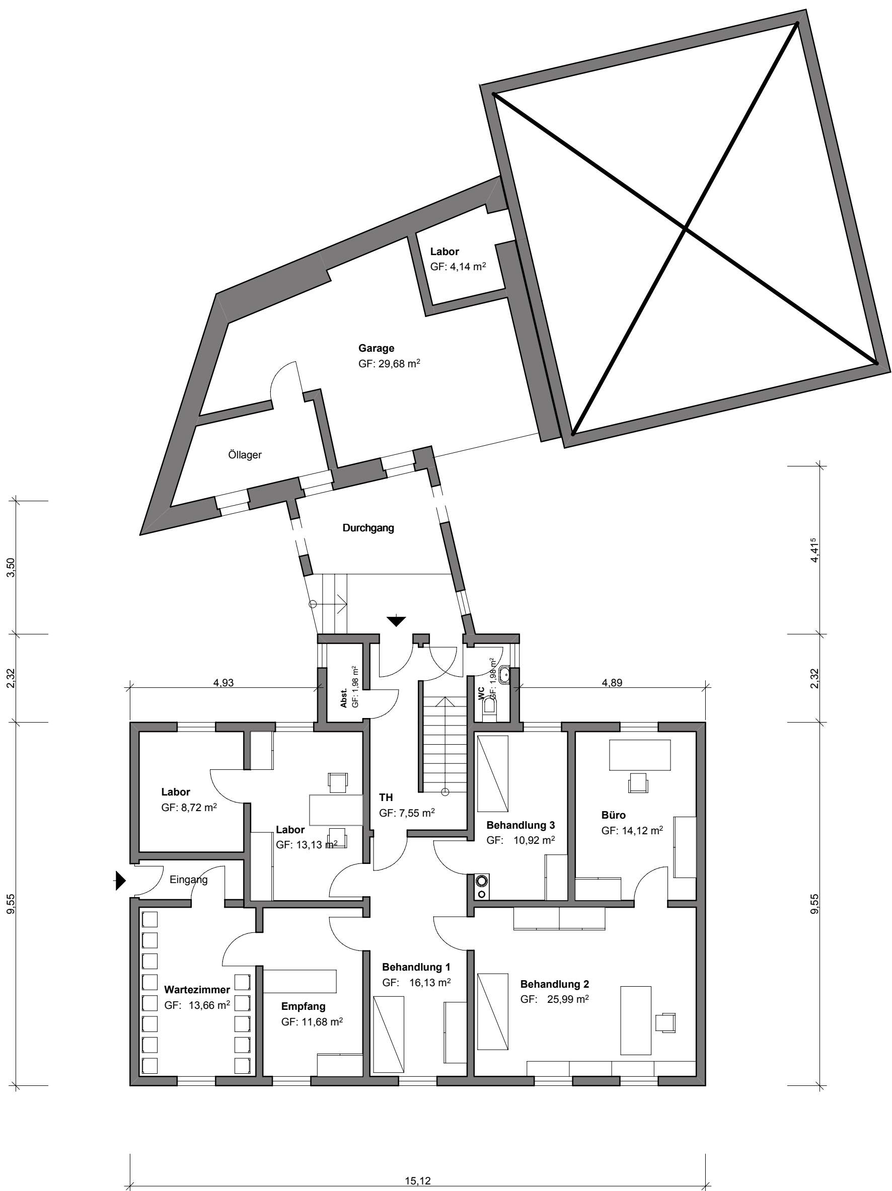
Grundriss Erdgeschoss
