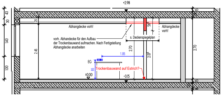
SCHNITT | M= 1:100
