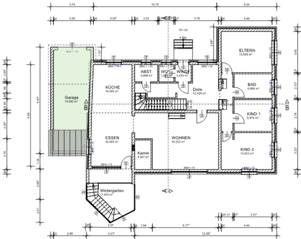
Grundriss EG
